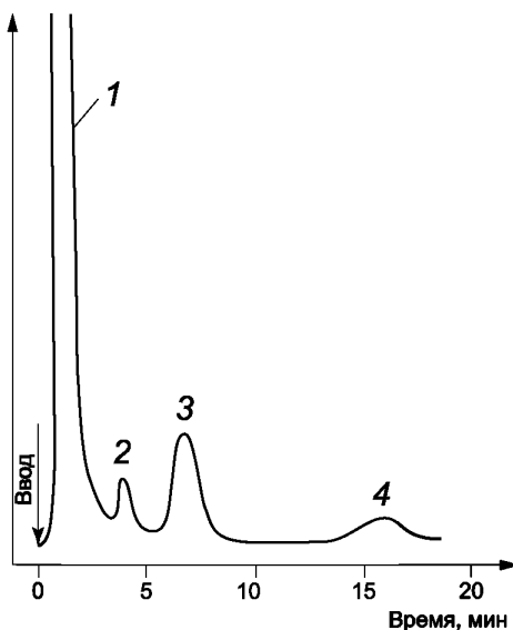
Рисунок 1 — Типовая хроматограмма этиленгликоля на колонке I
