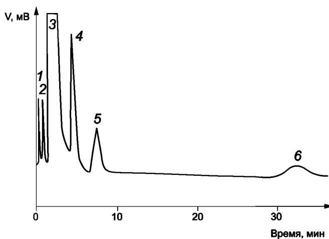
Рисунок 1 — Типовая хроматограмма этиленгликоля на колонке I
